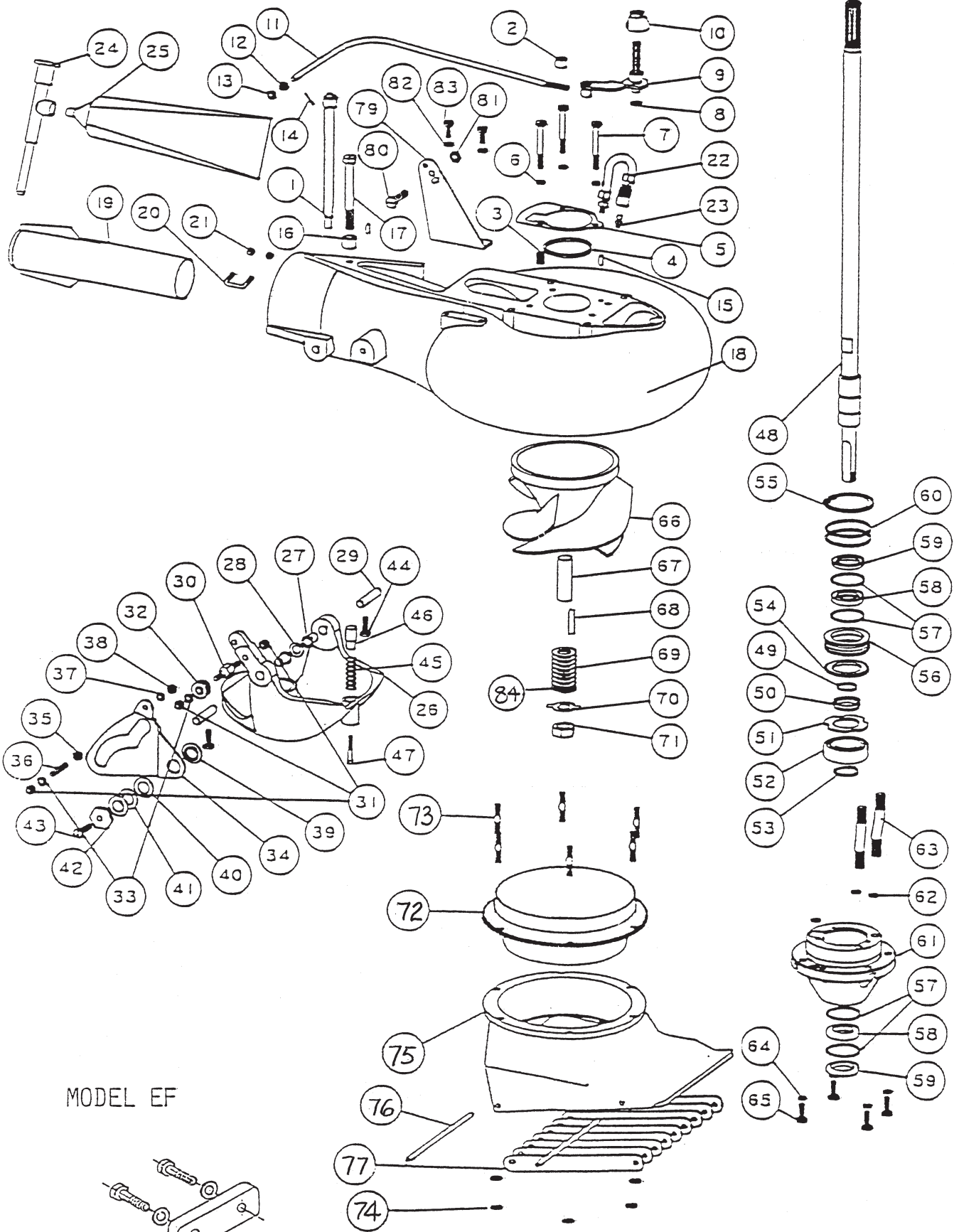
ANODE KIT 1693
